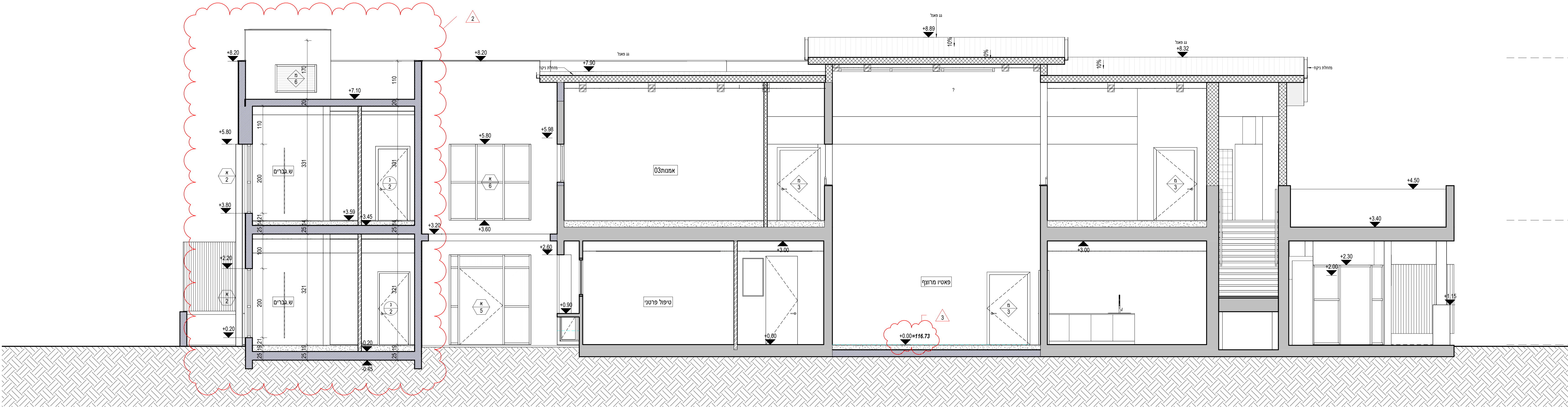
חתך ז-ז 1 : 50
