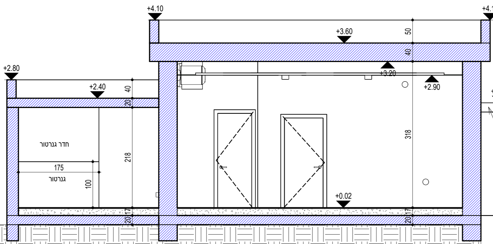
חתך ג-ג 1 : 50
