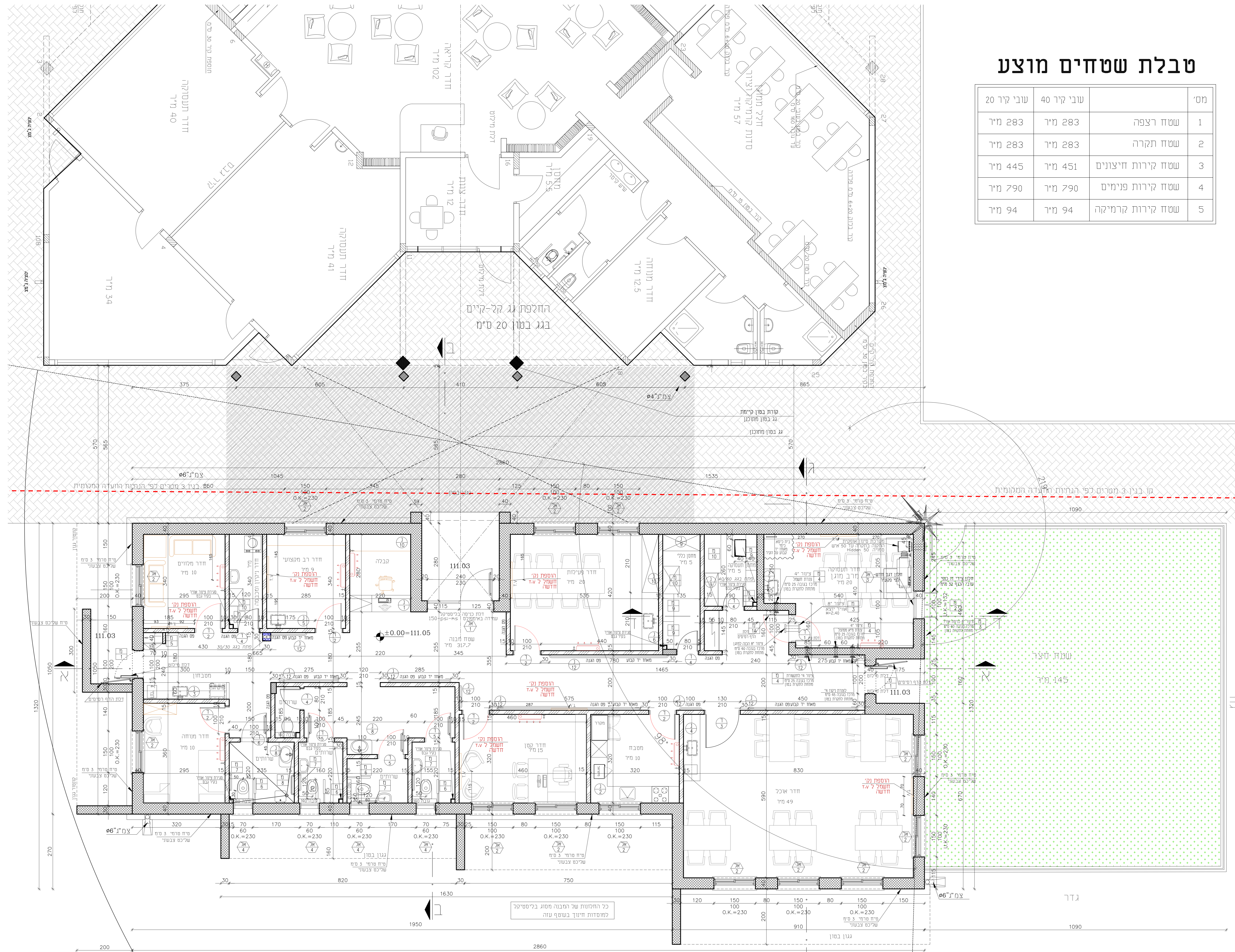
תכנית קומת קרקע ק.מ. 1:50
