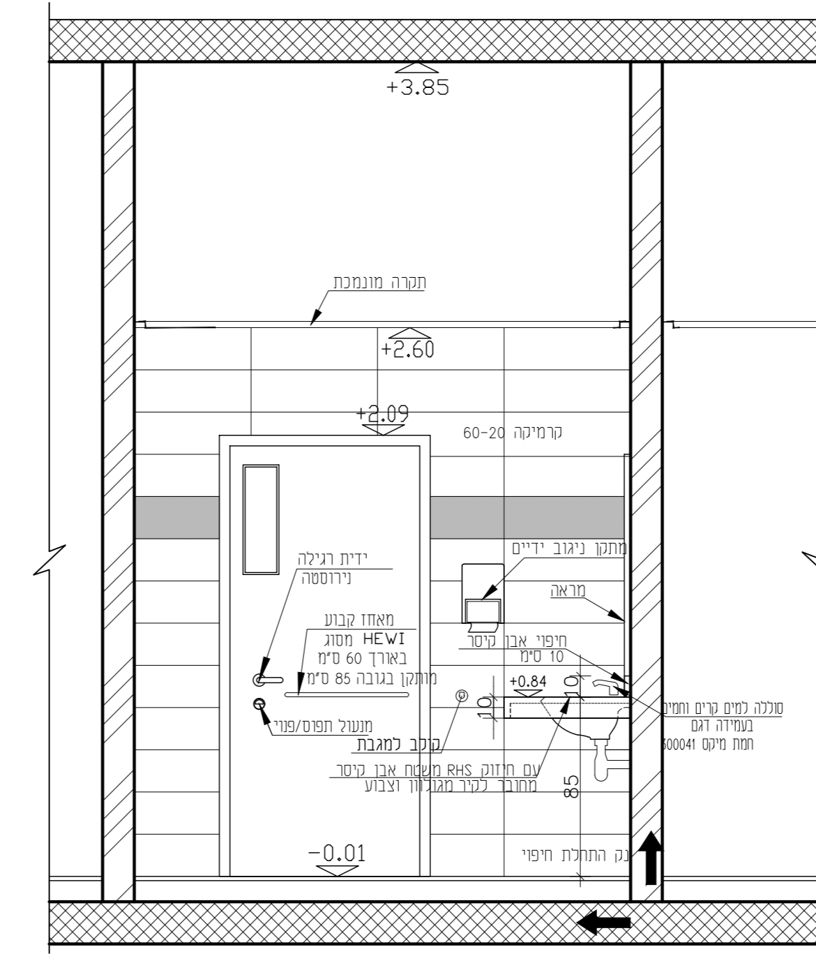
פריסות שרותי נכה. מבט 1 ק.מ.25:1
