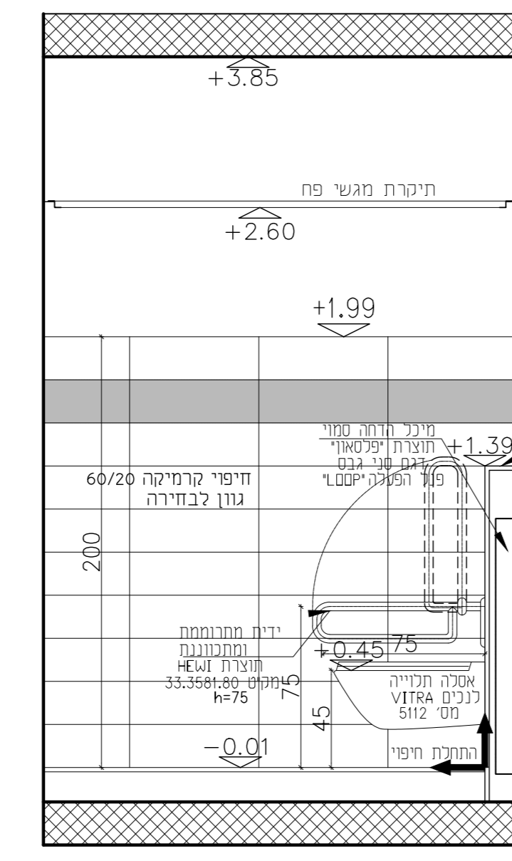
מבט 6 ק.מ.25:1
