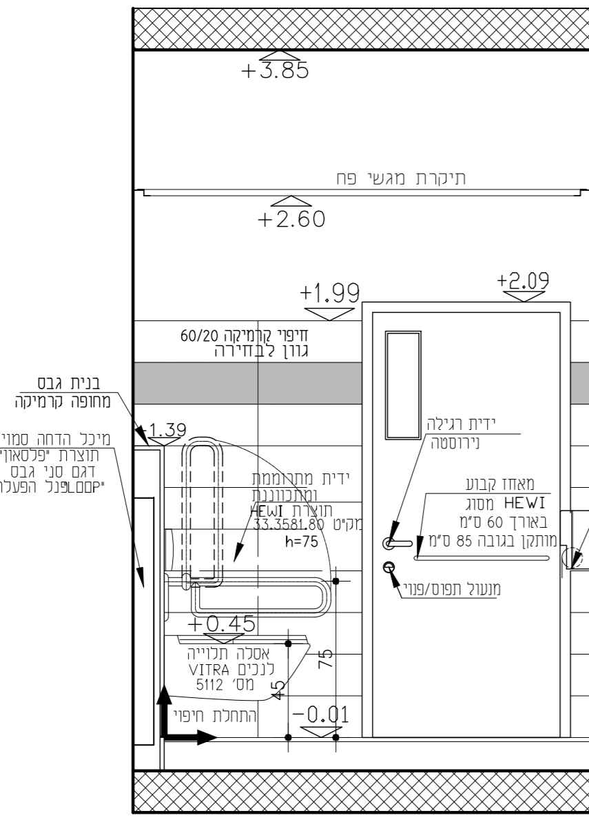
מבט 9 ק.מ.25:1
