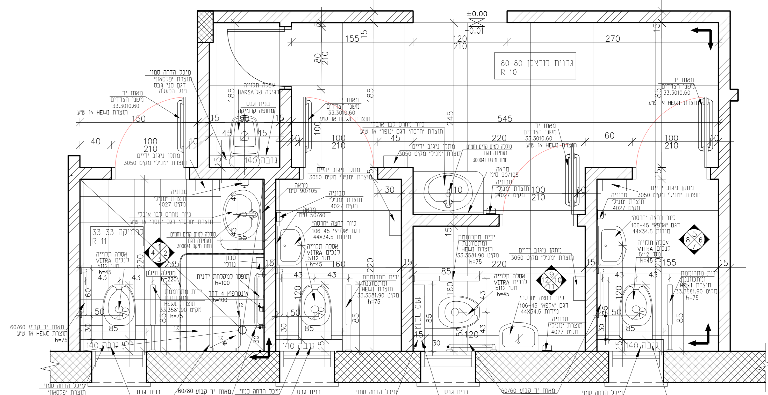
פריסות חדר שרותים תכנית ק.מ.25:1
