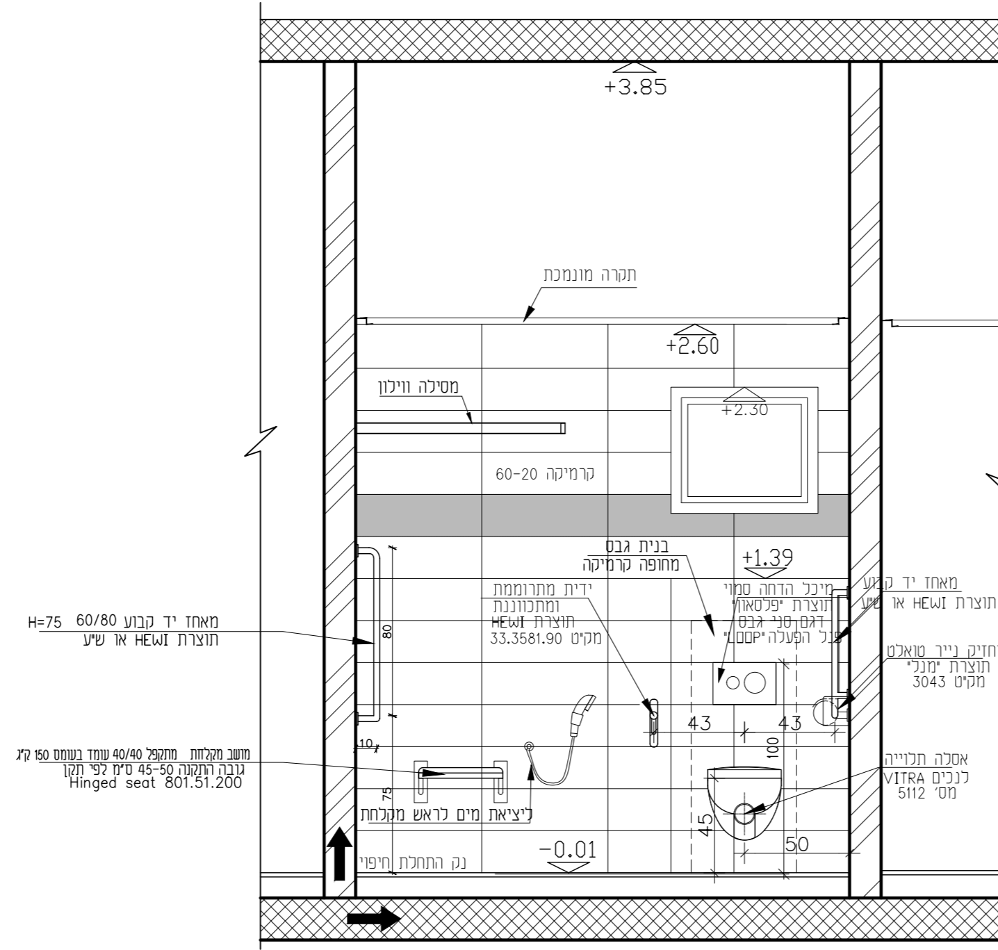
פריסות שרותי נכה. מבט 3 ק.מ.25:1
