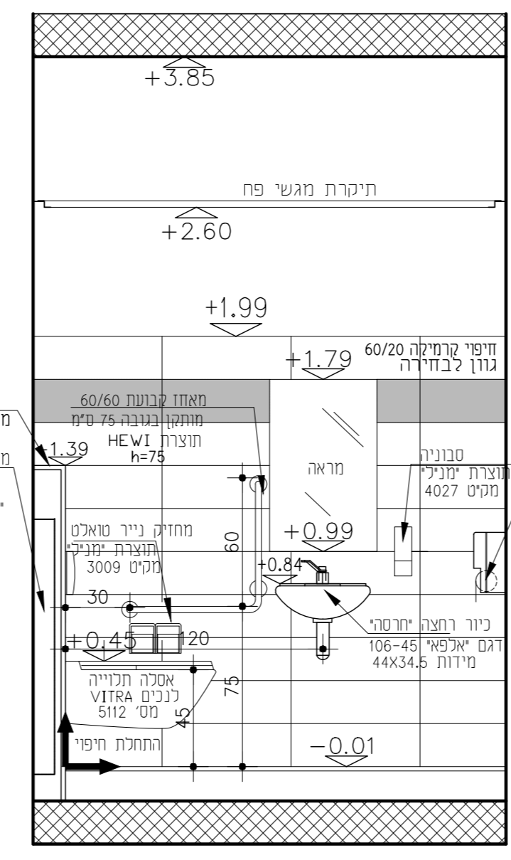
מבט 8 ק.מ.25:1
