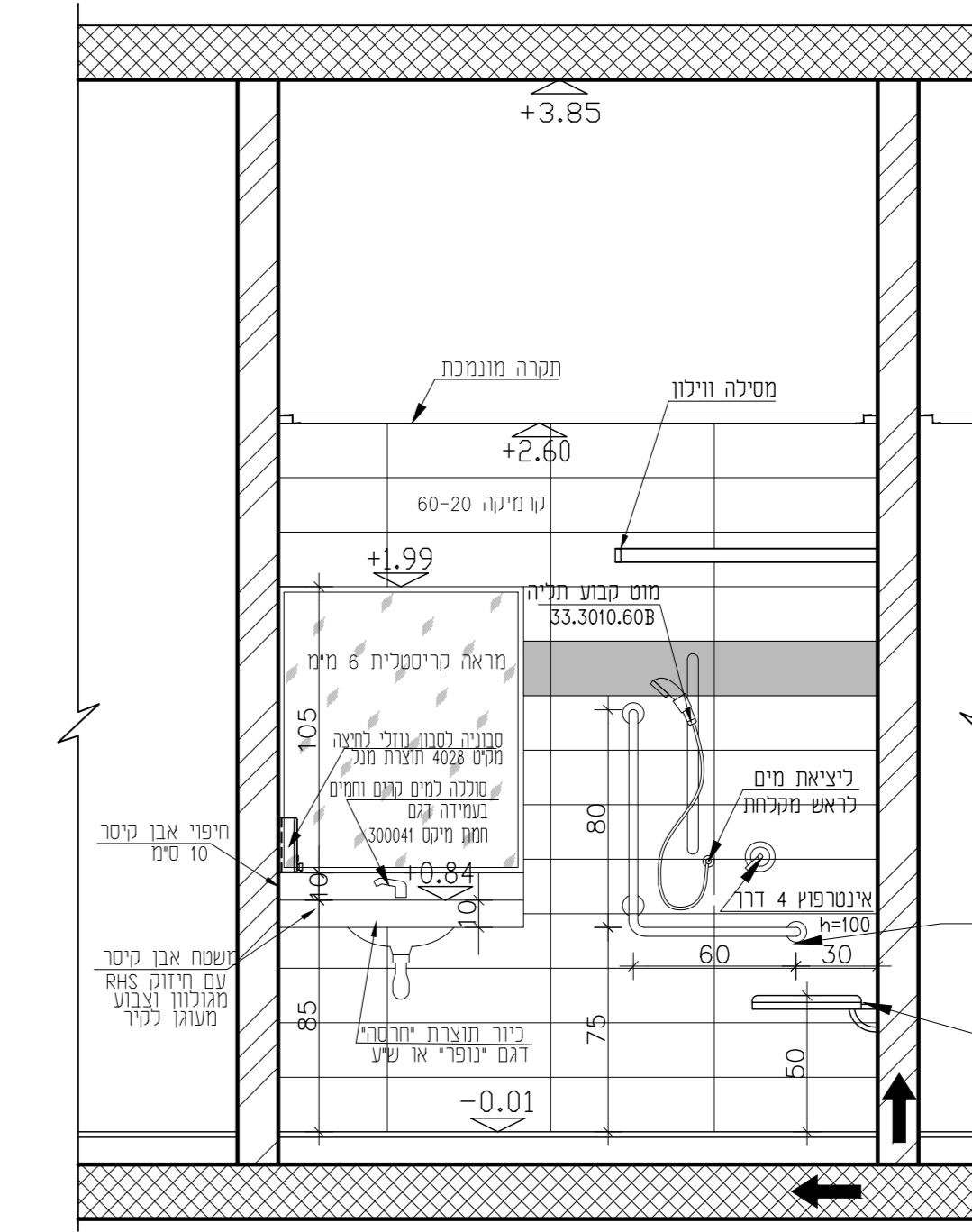
פריסות שרותי נכה. מבט 2 ק.מ.25:1
