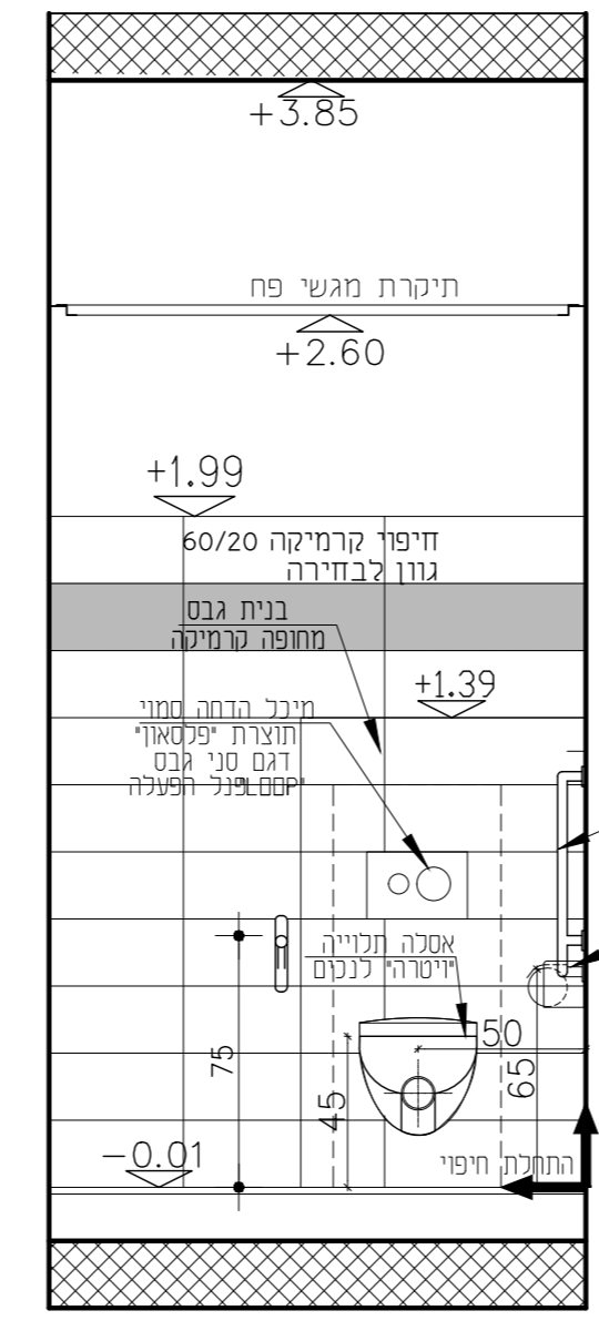
מבט 12 ק.מ.25:1
