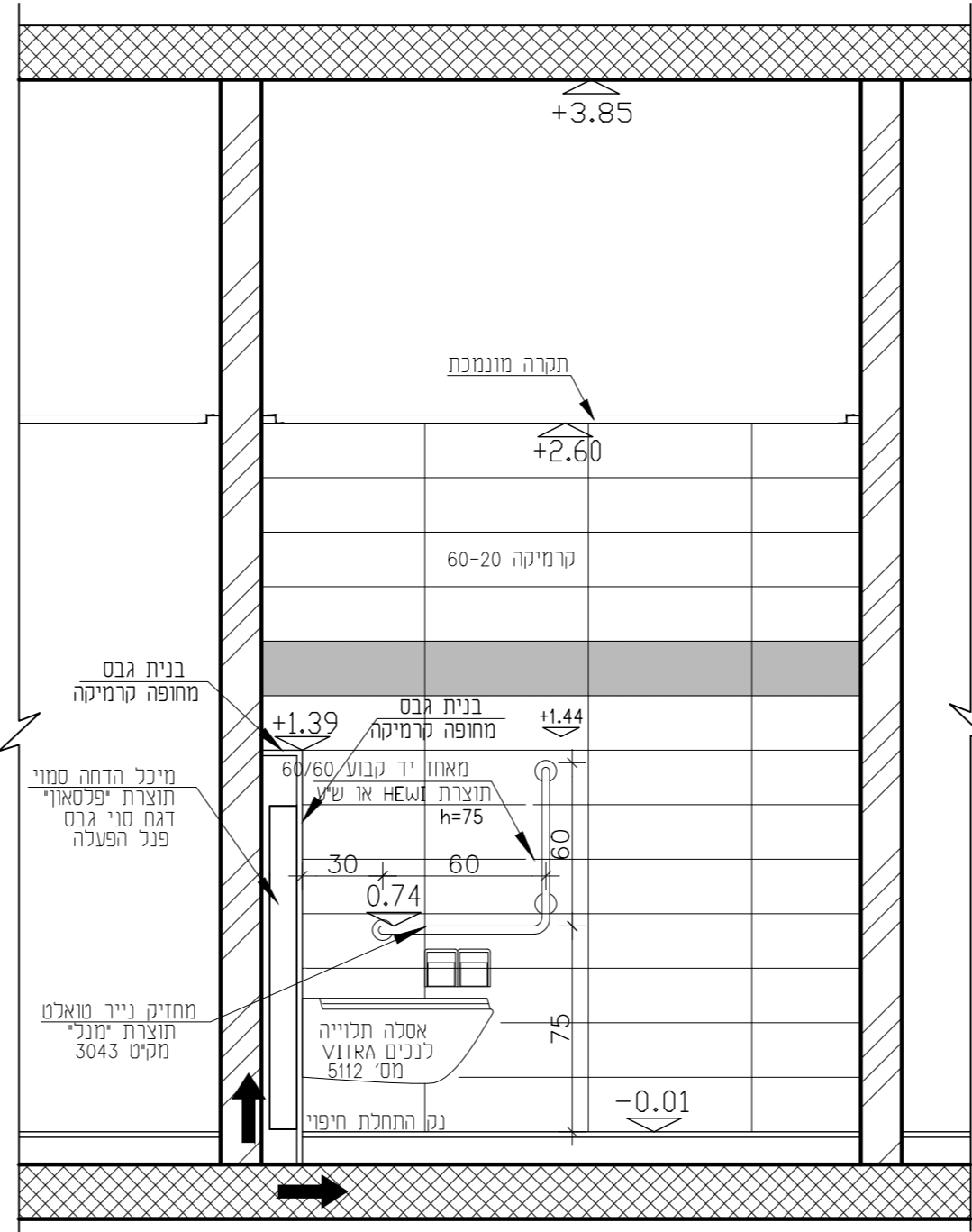
פריסות שרותי נכה. מבט 4 ק.מ.25:1
