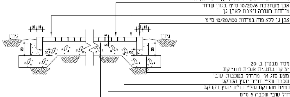
חתך 2-2. ק.מ. 1:20
