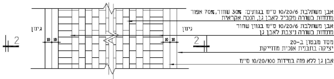
תכנית. ק.מ. 1:20
