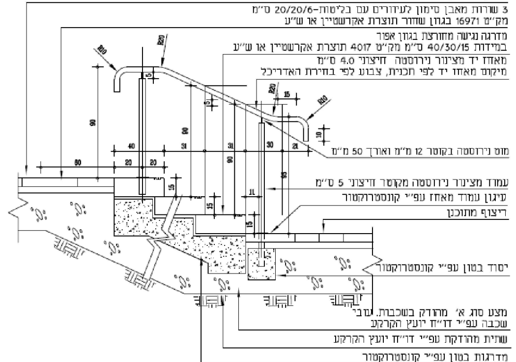
חתך 5-5 ק.מ. 1:20
