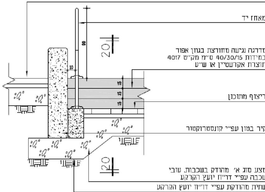
חזית 4-4 ק.מ. 1:20
