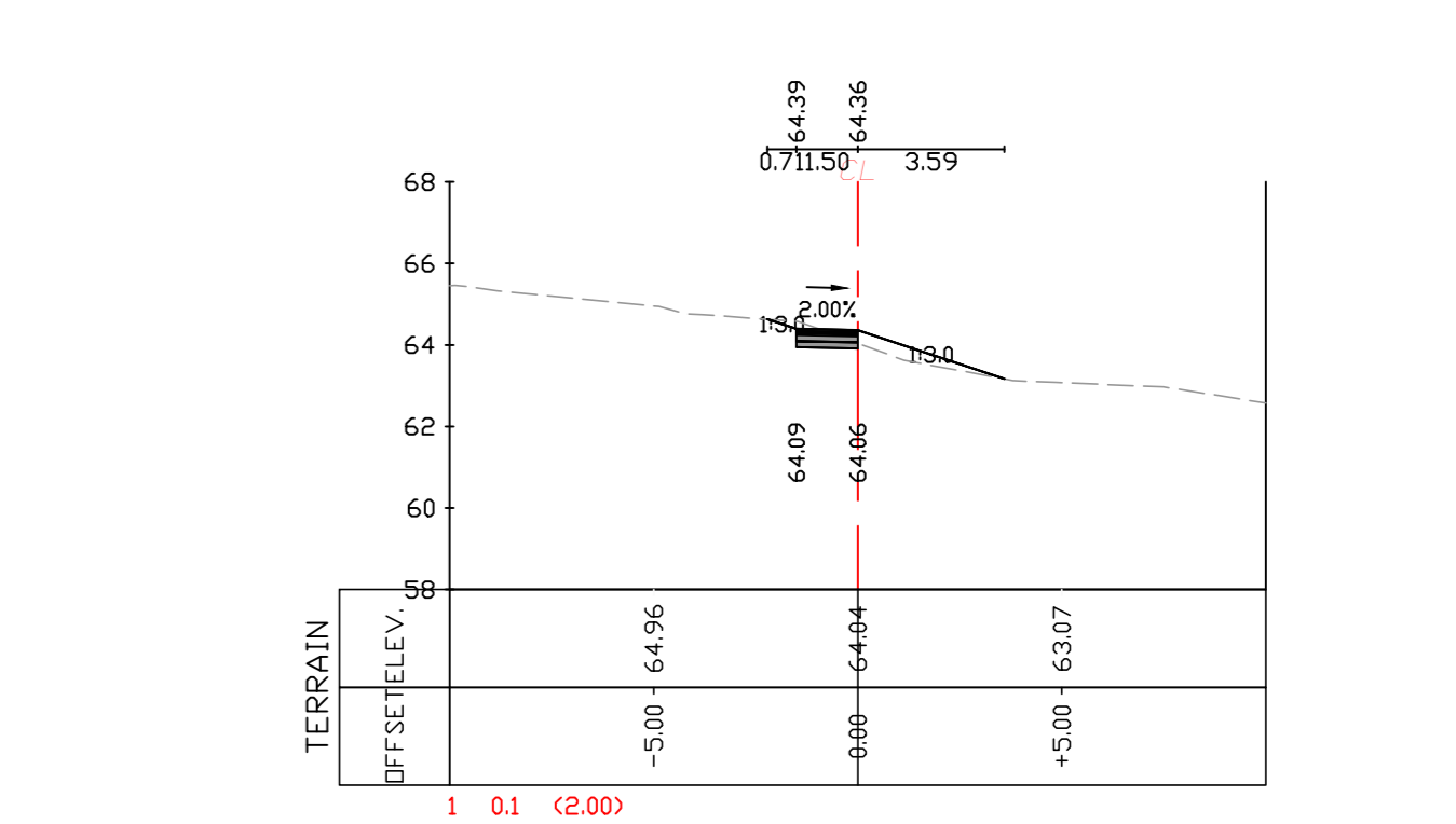
חתכים לרוחב בשביל קני"מ 1:200
