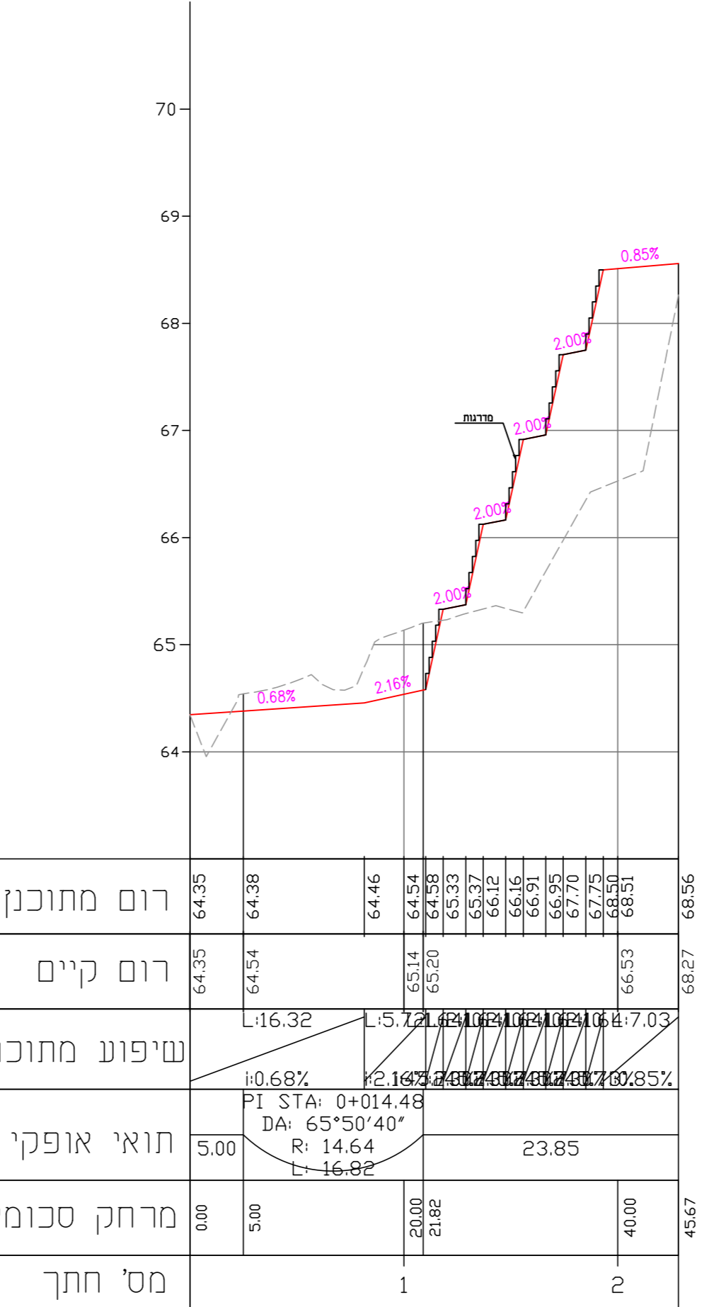
חתך באורך השביל קני"מ 1:500/50
