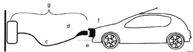
טעינת רכב חשמלי במצב פעולה 4:
