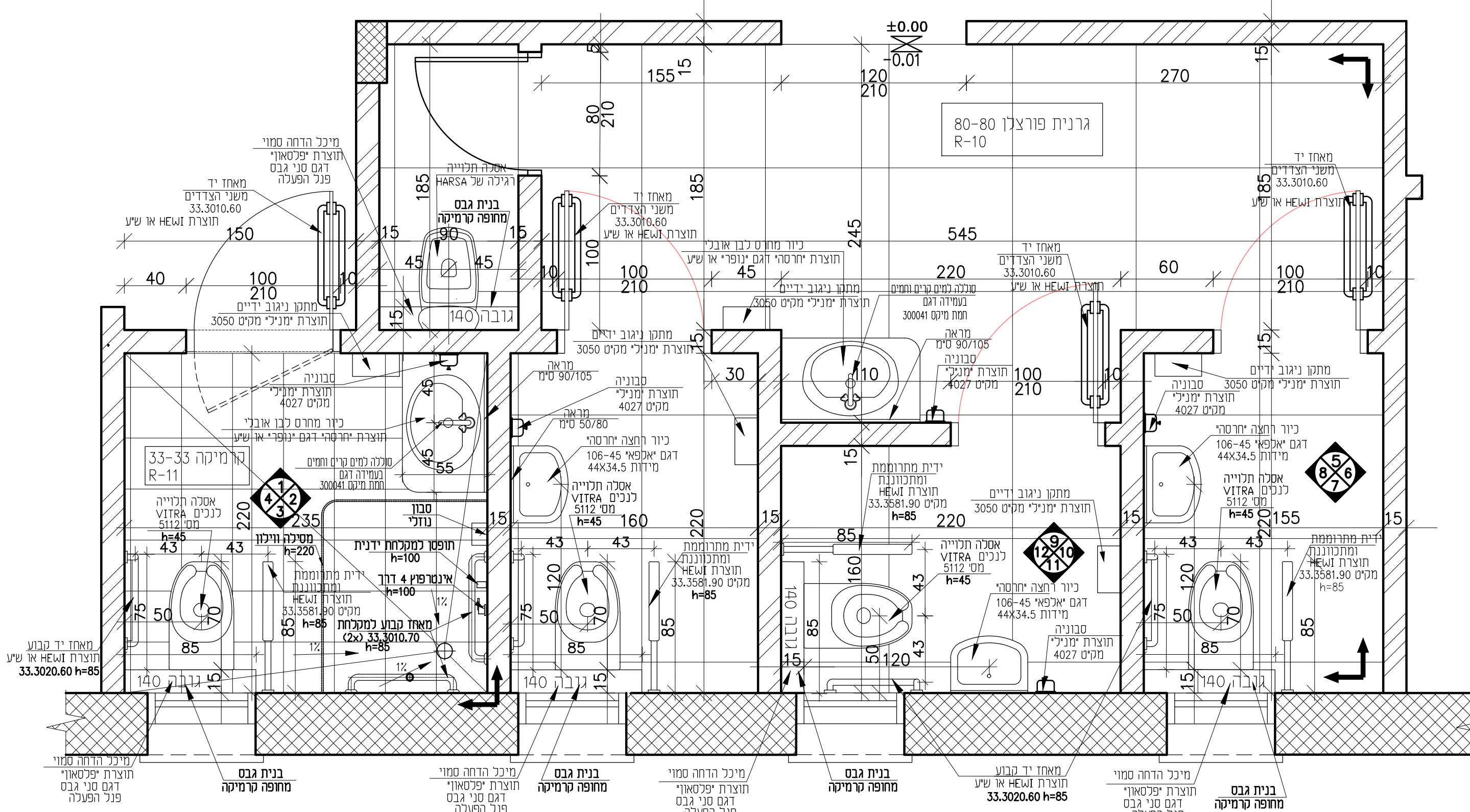
פריסות חדר שרותים תכנית ק.מ.25:1
