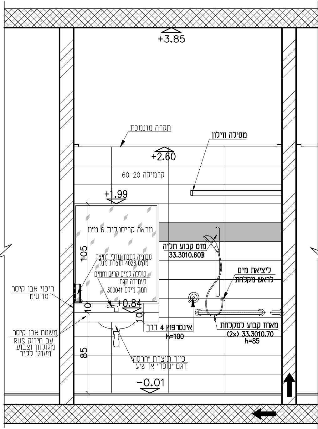
פריסות שרותי נכה. מבט 2 ק.מ. 1:25
