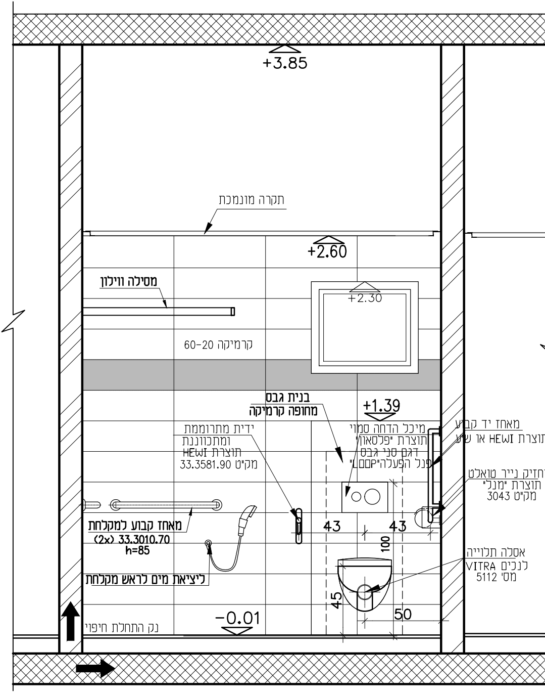
פריסות שרותי נכה. מבט 3 ק.מ. 1:25
