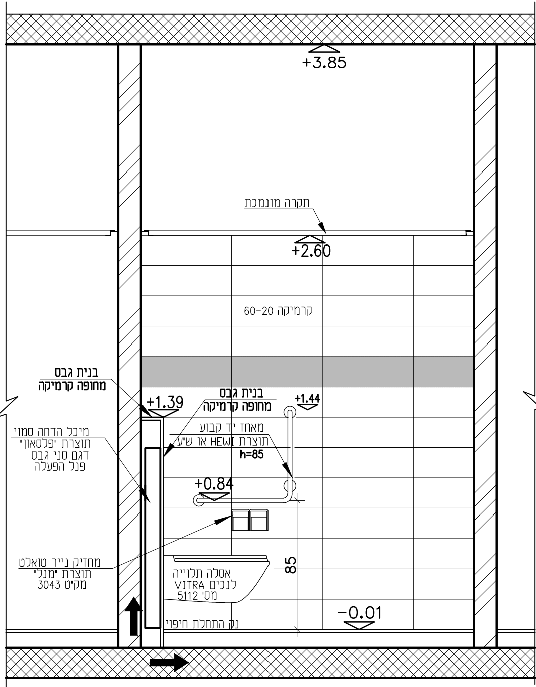
פריסות שרותי נכה. מבט 4 ק.מ. 1:25
