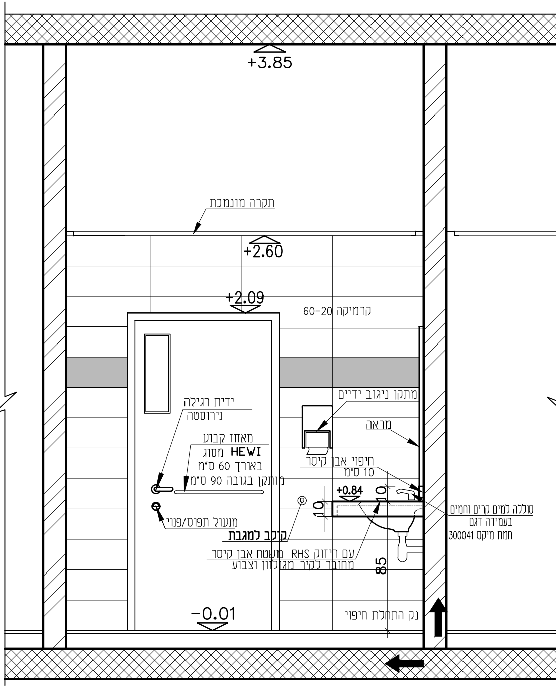
פריסות שרותי נכה. מבט 1 ק.מ.25:1
